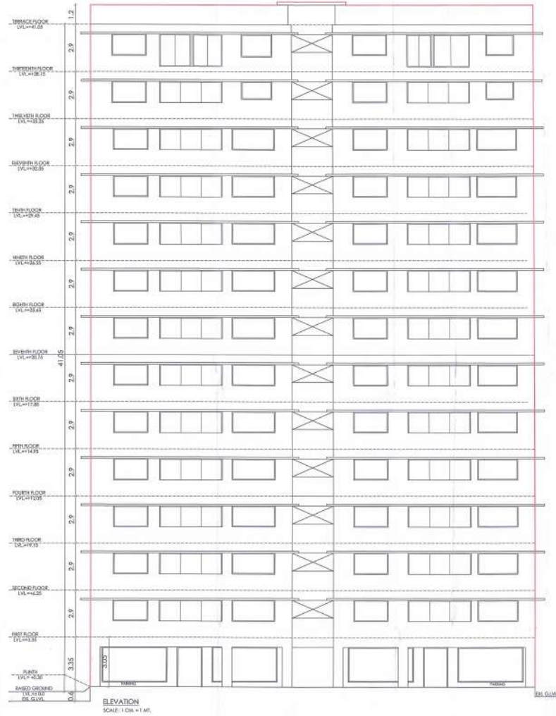
ELEVATION SCALE: 1 CM = 1 MT.
