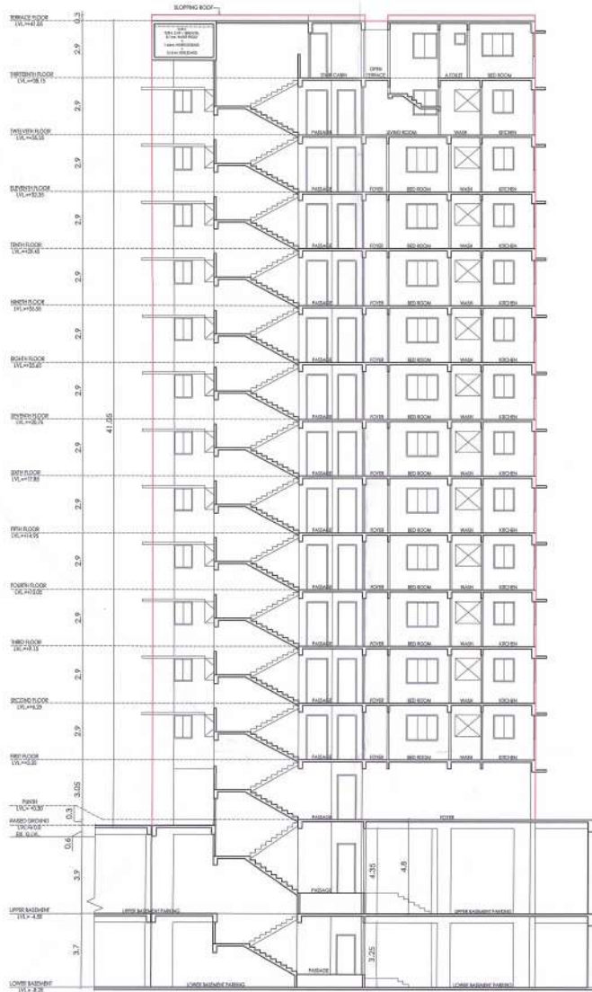
SECTION AA SCALE: 1 CM = 1 M
