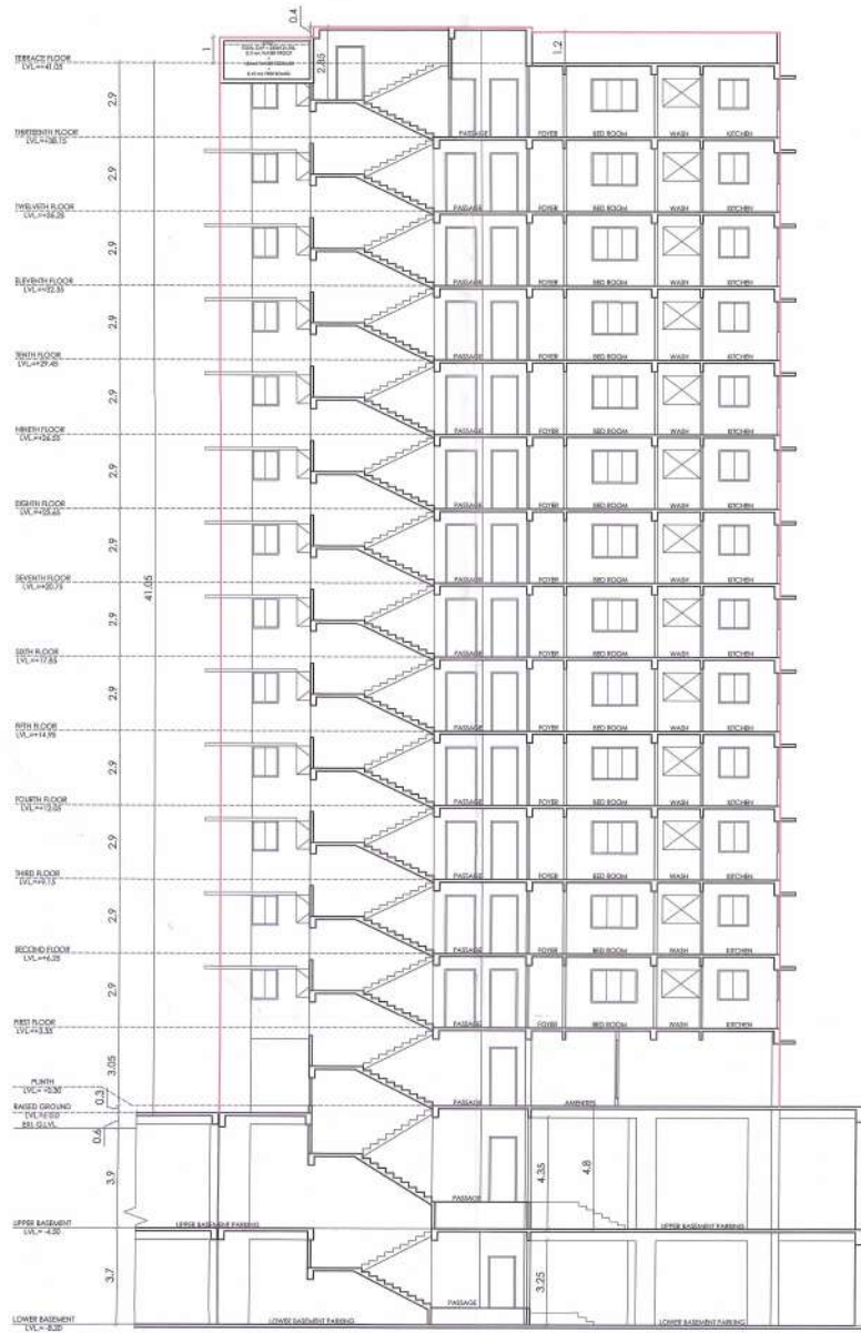
SECTION-AA SCALE: 1 CM = 1 MT.
